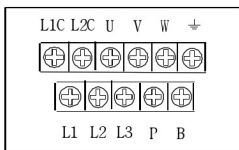
[ EDA7015 ~ EDA7045 주회로 단자대 ]
