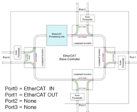
[[IN/OUT 포트 터미널과 ESC (EtherCAT Slave Controller)의 결선상태]
