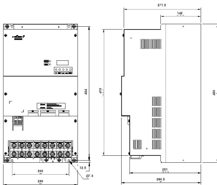
[ 외형도 F ]
