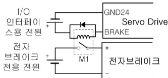
[출력 접점 배선방법(예), I/O 인터페이스용 전원 ≠ 전자 브레이크 전용 전원]
