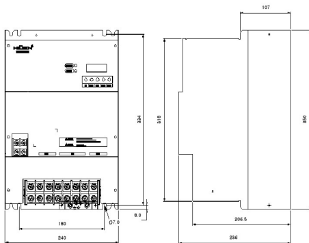
[ 외형도 E ]
