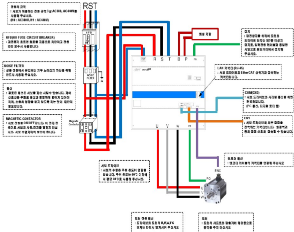
[주변 기기의 접속 예 (EDA7550)]
