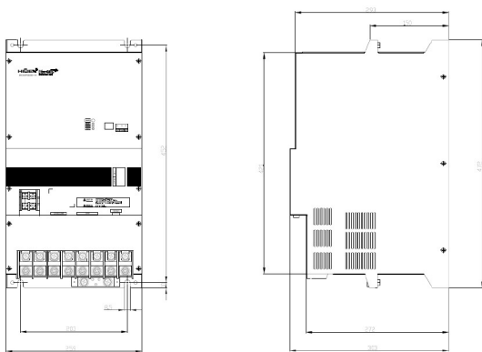
[ 외형도 1 ]
