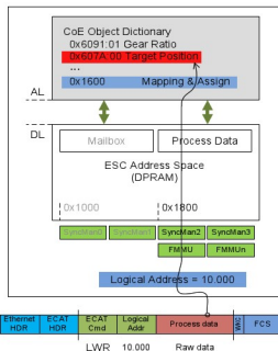
[FMMU 의 논리 주소 (PDO Access)]
