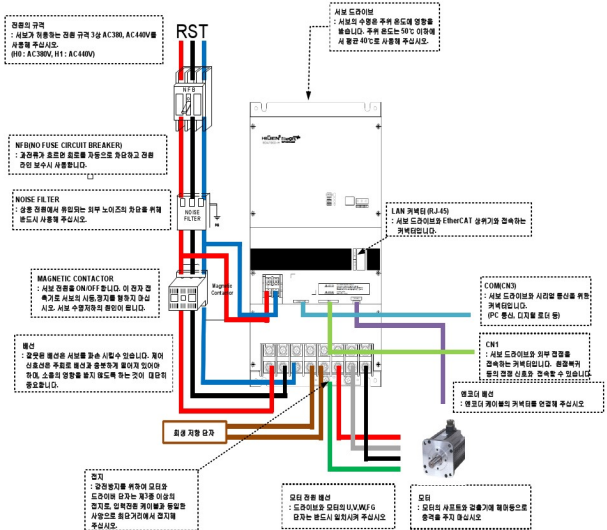
[주변 기기의 접속 예 (EDA7150)]
