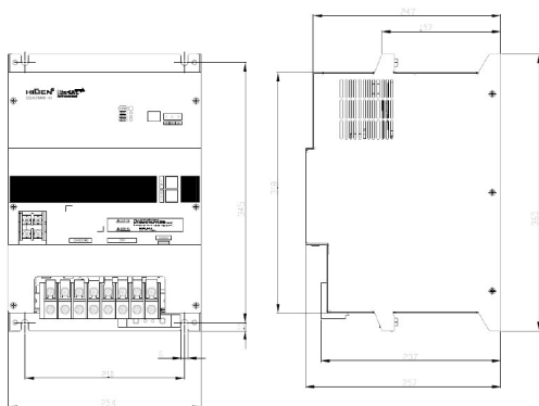
[ 외형도 H ]
