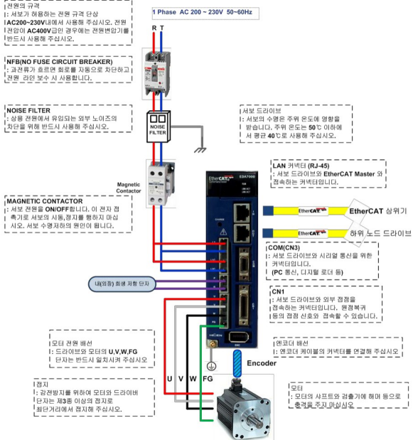
[주변 기기의 접속 예 (EDA7001, EDA7002)]
