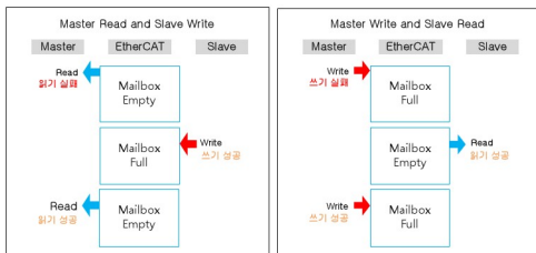
[SyncManager 메일박스 모드]
