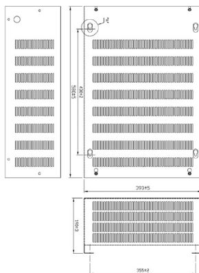
[회생저항 외형도 D, 단위(mm)]
