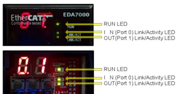
[EtherCAT 표시 LED 및 Node 디스플레이]
