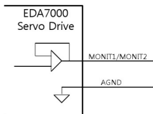
[아날로그 출력 신호 배선방법(예)]
