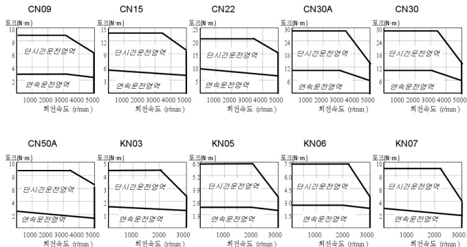
토크 - 속도 특성
