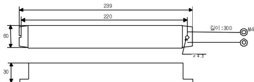
[회생저항 외형도 A, 단위[mm]]
