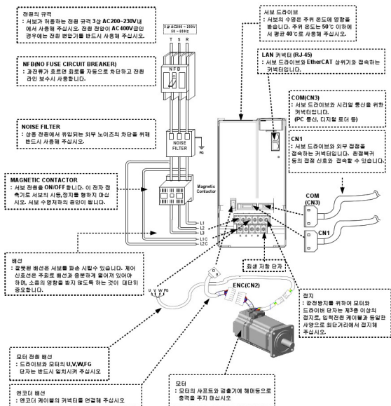
[주변 기기의 접속 예 (EDA7045)]
