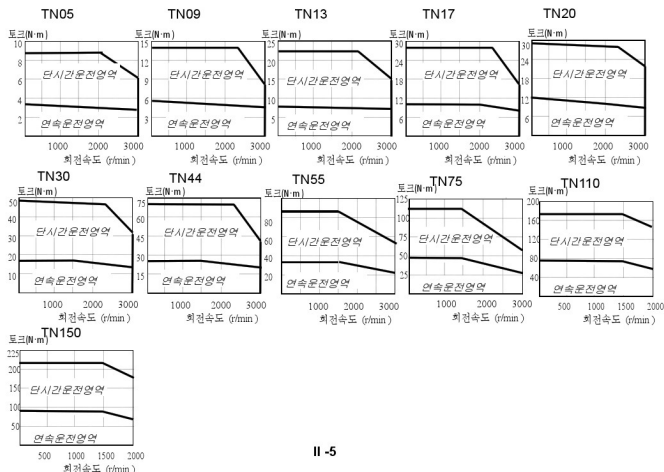
토크 - 속도 특성
