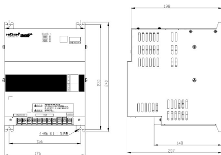
[ 외형도 G ]
