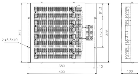
[회생저항 외형도 B, 단위(mm)]
