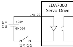
[입력 점점 배선방법(예)]
