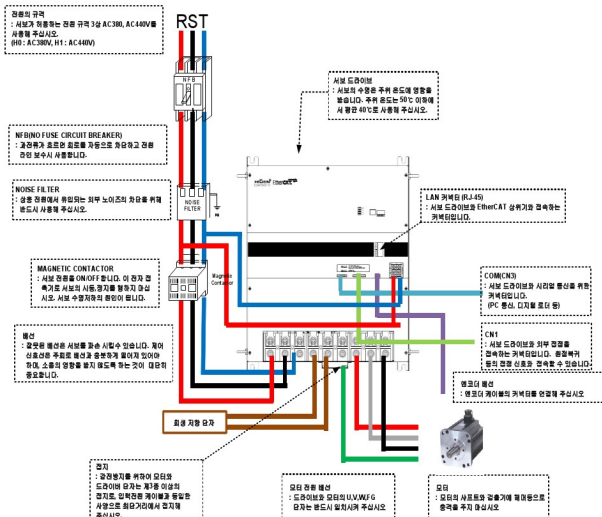
[주변 기기의 접속 예 (EDA7370)]
