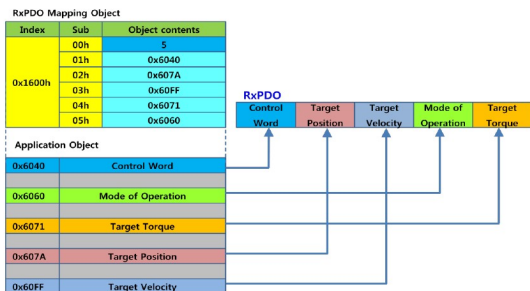
[1st. RxPDO 맵핑 예]
