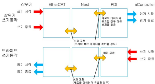
[SyncManager 버퍼 모드]
