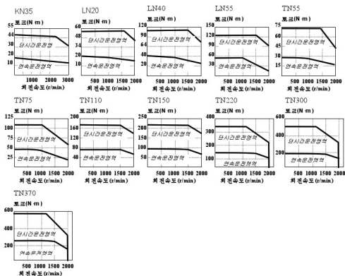
토크 - 속도 특성
