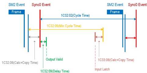
[Sync0 이벤트에 대한 로컬 사이클 동기]
