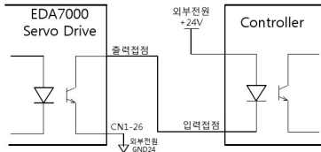
[출력 접점 배선방법(예)]
