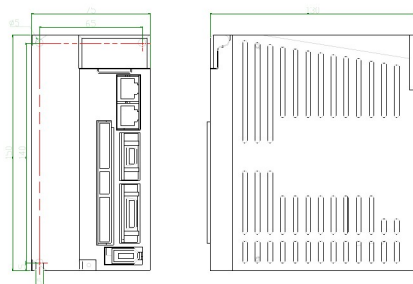
[ 외형도 B ]
