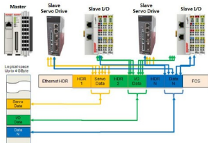
[논리 주소 (Logical Address Image)]
