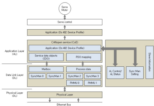
[EtherCAT(CoE) 슬레이브 디바이스 아키텍처]
