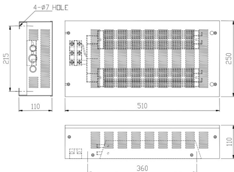
[회생저항 외형도 C, 단위(mm)]
